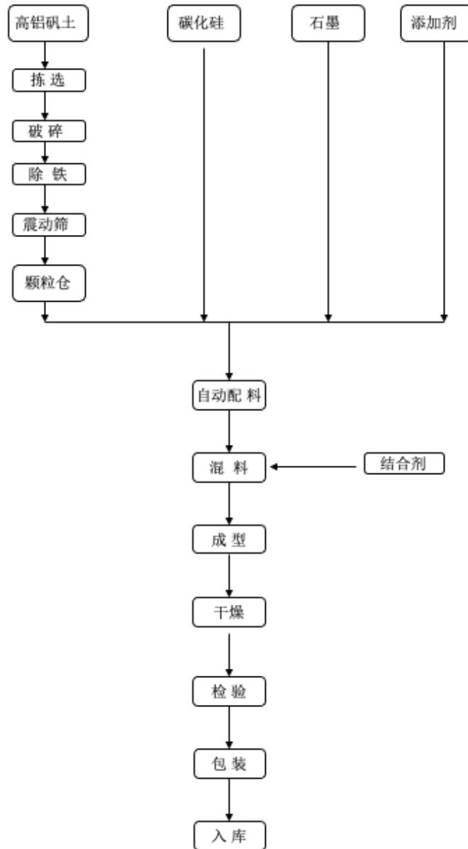
图 1-1 耐火砖生产工艺流程图
