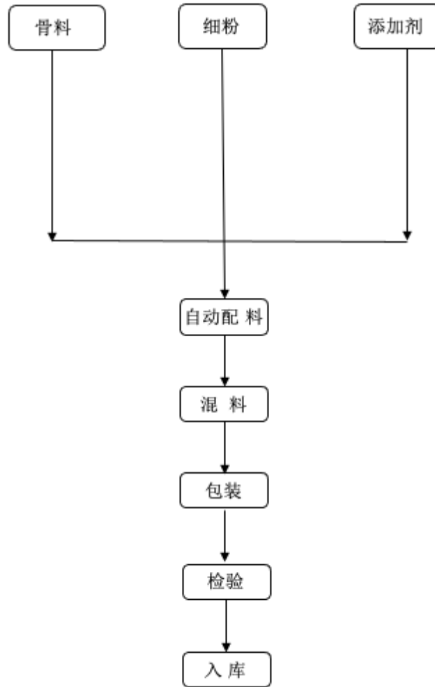
图 1-2 不定形浇注料生产线生产工艺流程图
